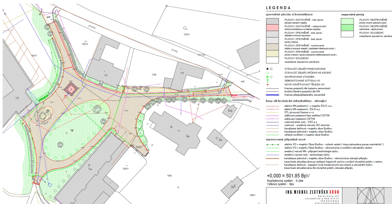
Obr. 5 výřez z výkresu C.3 situace koordinační, příloha žádosti
