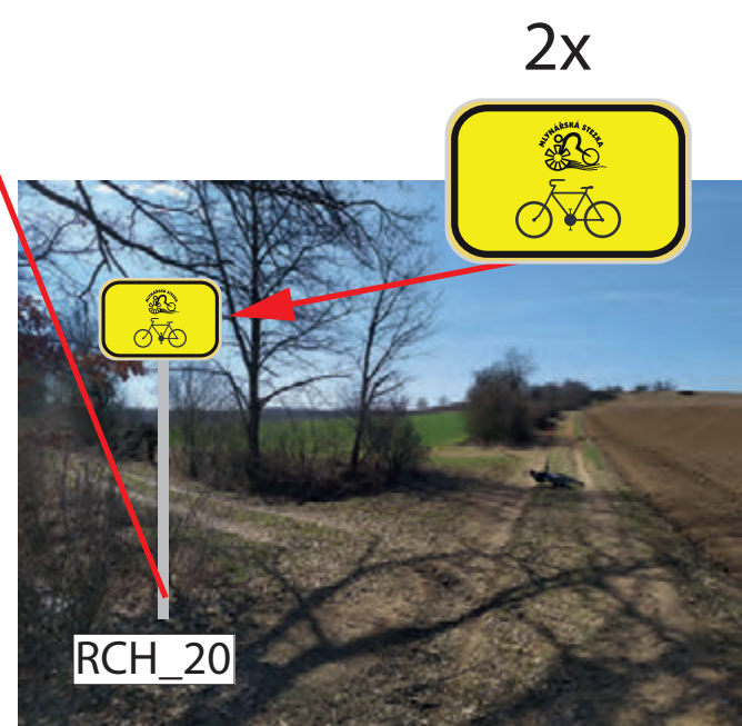
INSTALACE 2x IS21a (MLYNÁŘSKÁ) NA NOVÝ SLOUPEK SPOLEČNÝ PRO OBA SMĚRY V ZEMNÍ BETONOVÉ PATCE POZEMEK: PARC. Č. 1254/2 K. Ú. ROUCHOVANY (OBEC ROUCHOVANY)
