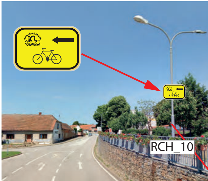
INSTALACE IS21b (MLYNÁŘSKÁ) NA SLOUP VEŘEJNÉHO OSVĚTLENÍ
