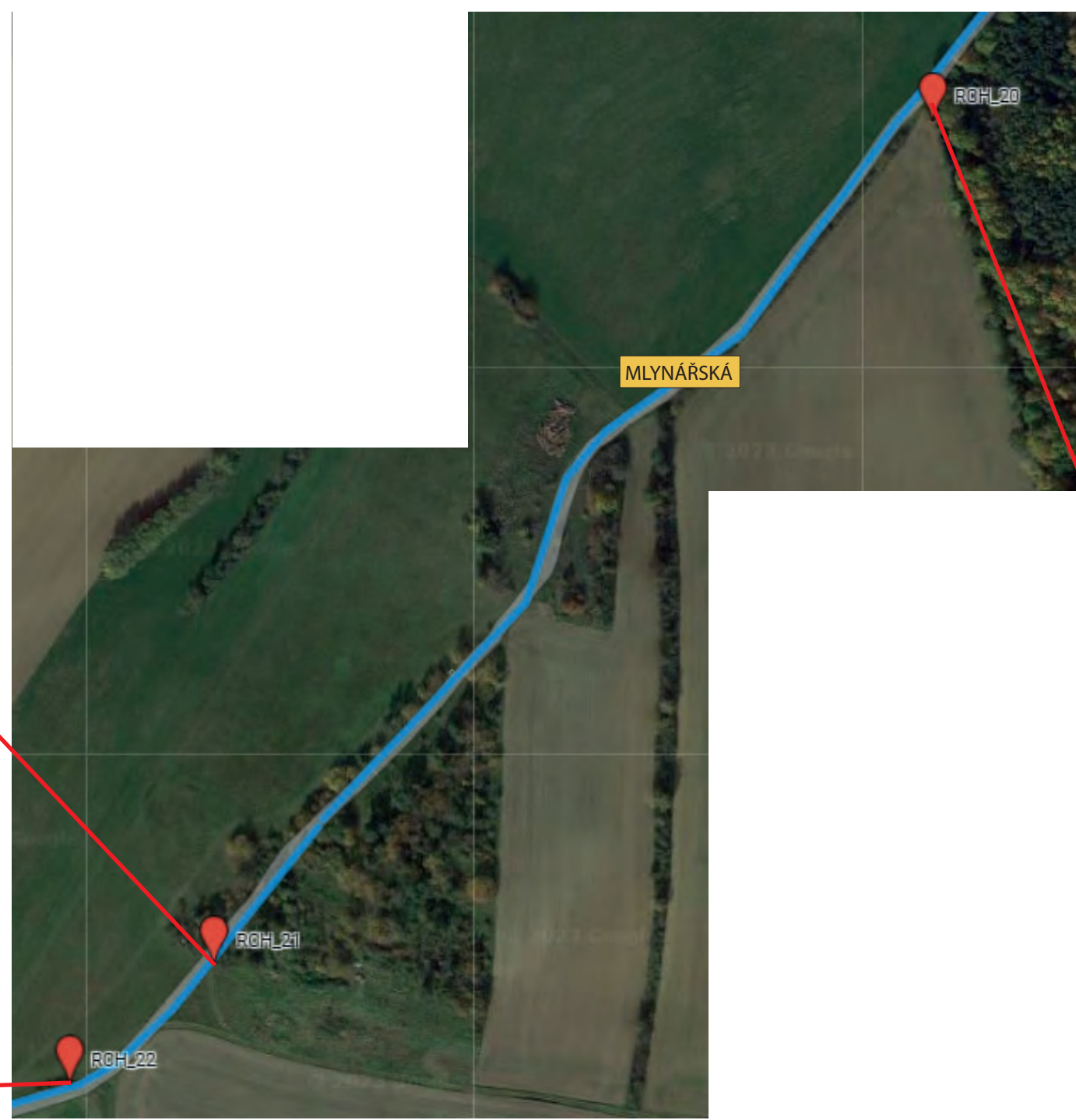
INSTALACE 2x IS21a (MLYNÁŘSKÁ) NA NOVÝ SLOUPEK SPOLEČNÝ PRO OBA SMĚRY V ZEMNÍ BETONOVÉ PATCE POZEMEK: PARC. Č. 1254/2 K. Ú. ROUCHOVANY (OBEC ROUCHOVANY)
