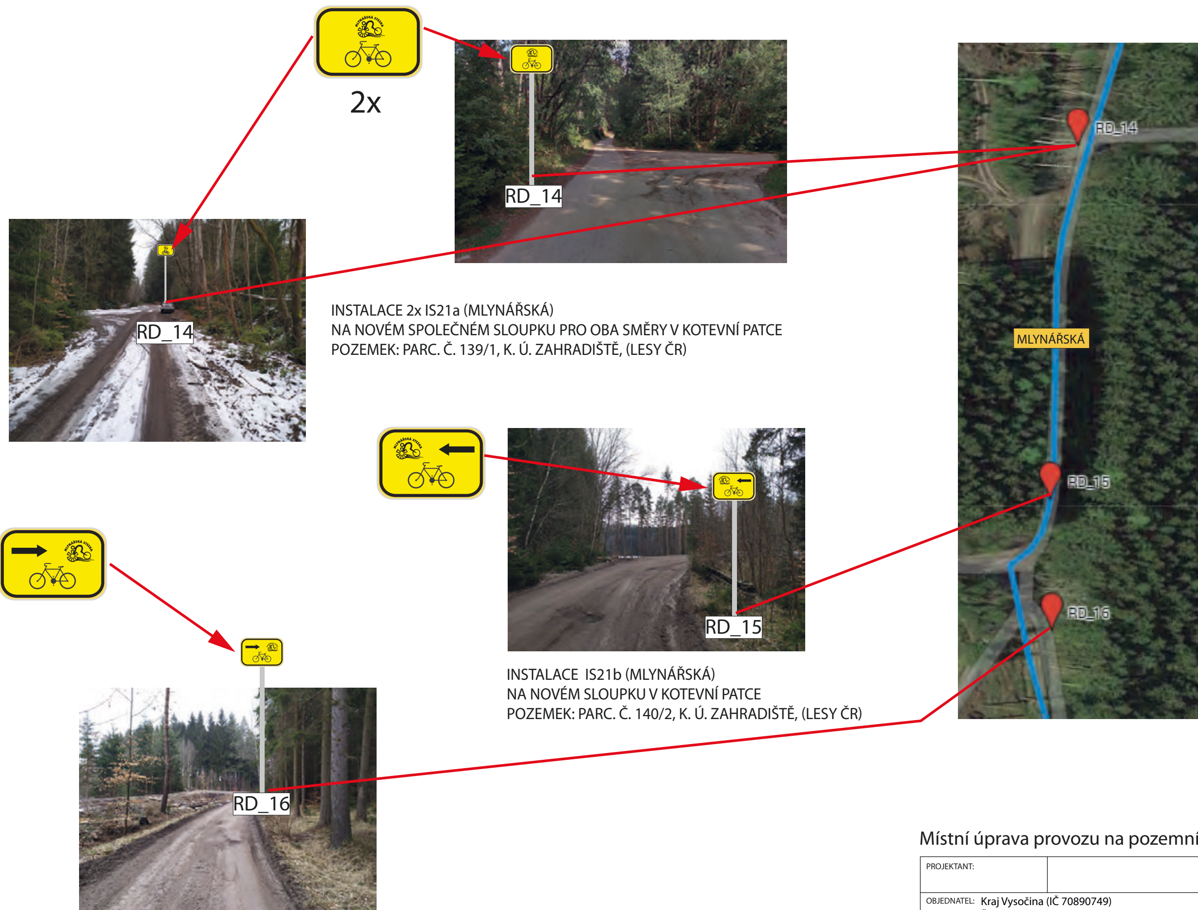
INSTALACE IS21c (MLYNÁŘSKÁ) NA NOVÉM SLOUPKU V KOTEVNÍ PATCE POZEMEK: PARC. Č. 140/2, K. Ú. ZAHRADIŠTĚ, (LESY ČR)
