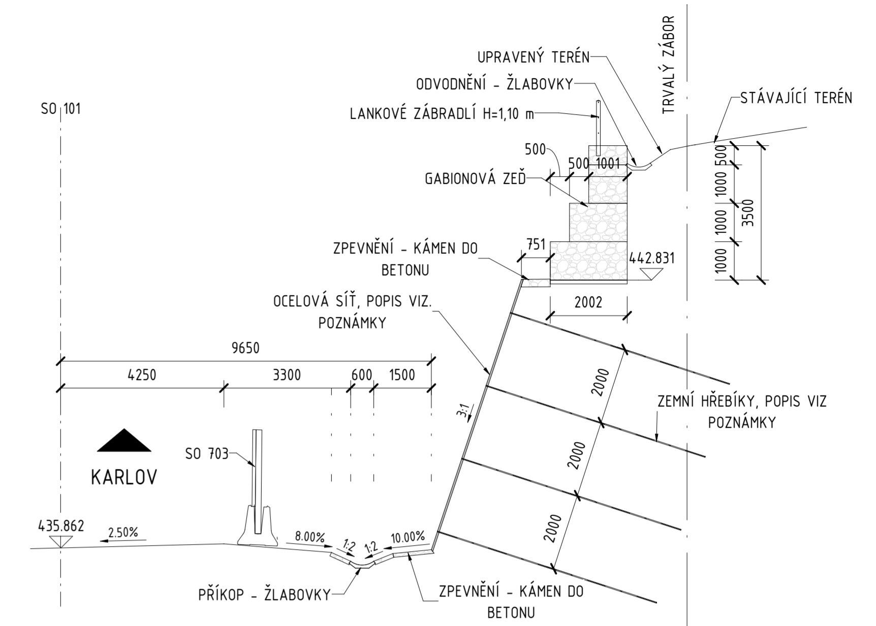
ŘEZ 1 1 : 100
