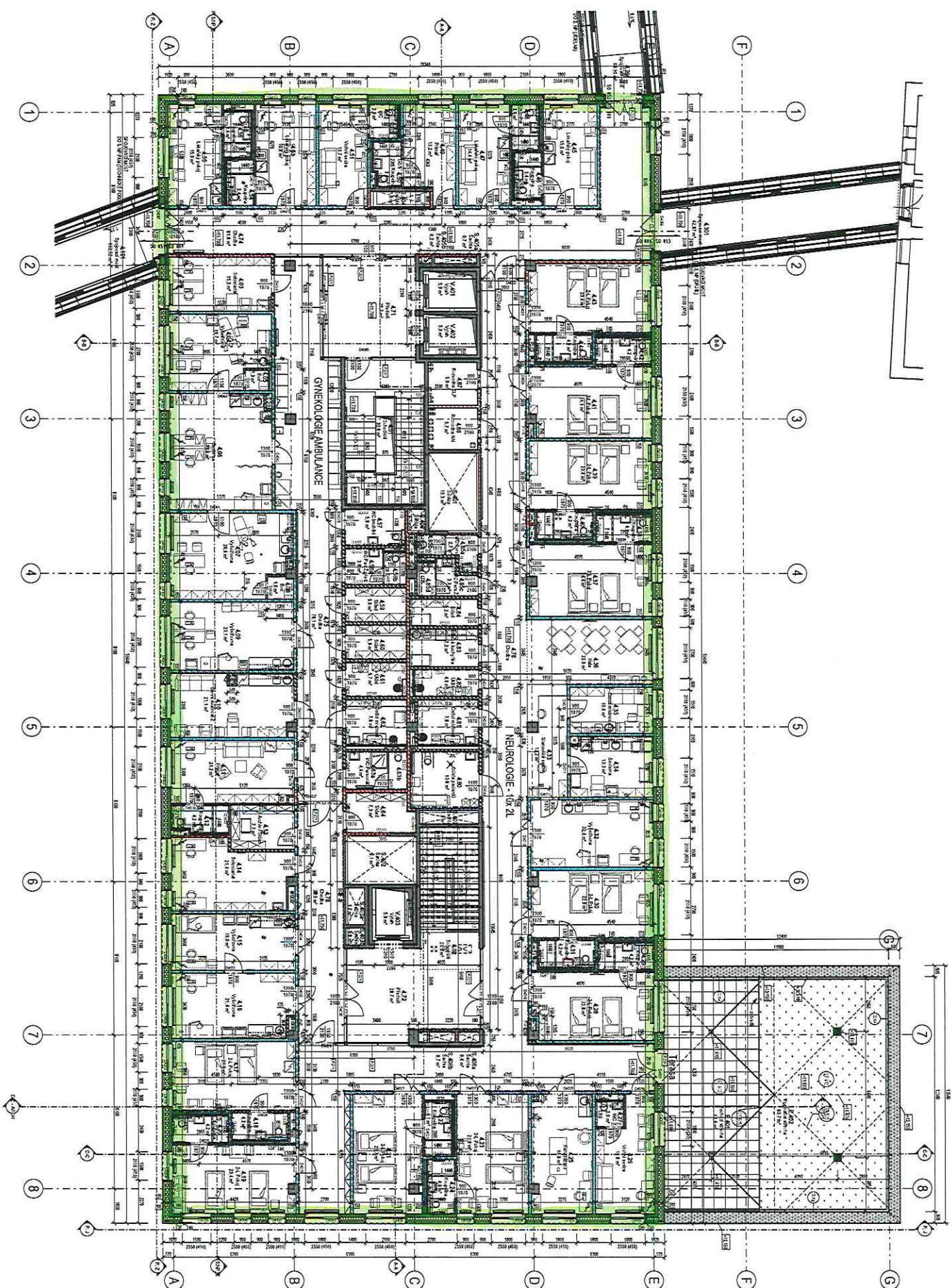
Půdorys 4. Nadzemního podlaží
