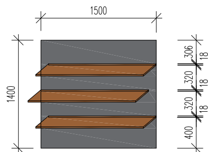
A16 -NÁSTĚNNÝ POLICOVÝ PANEL
