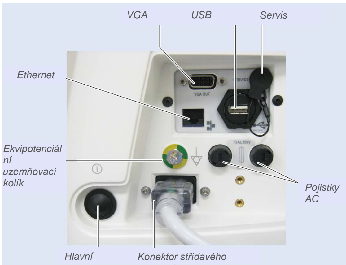
Obr. 11 Popis Automatizovaného kontroléru – Zadní část
