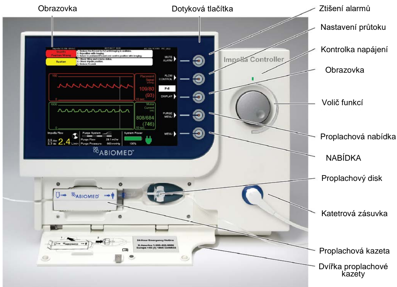
Obr. 10 Popis Automatizovaného kontroléru – přední část
